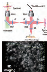
2 単一対物レンズ光シート顕微鏡 Single objective light sheet μ-scopic by APOM
