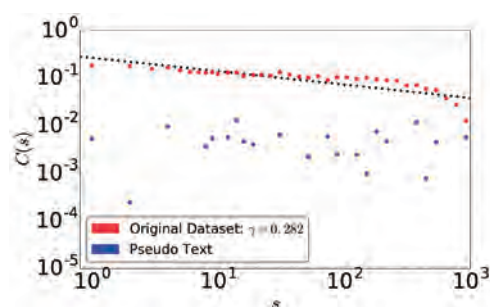
1 文字レベル深層言語モデルには長期記憶がない (赤が実データ、青が深層学習) Character-based deep learning has no long memory
