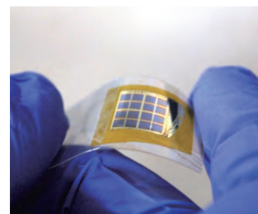
③ ELO法により作製した薄膜太陽電池 Thin-film solar cells by developed with ELO technique
