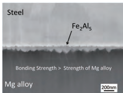
② ナノレベルの金属間化合物で実現した鋼/Mg合金の 強固な結合 Strong steel/Mg alloy bonding by ultra-thin intermetallic compound
