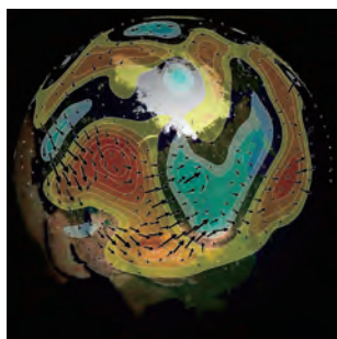
1 2010年8月に日本に記録的猛暑をもたらした上空の高・低気圧の波動 Wavy pressure anomalies caused a heat wave to Japan in August 2010
