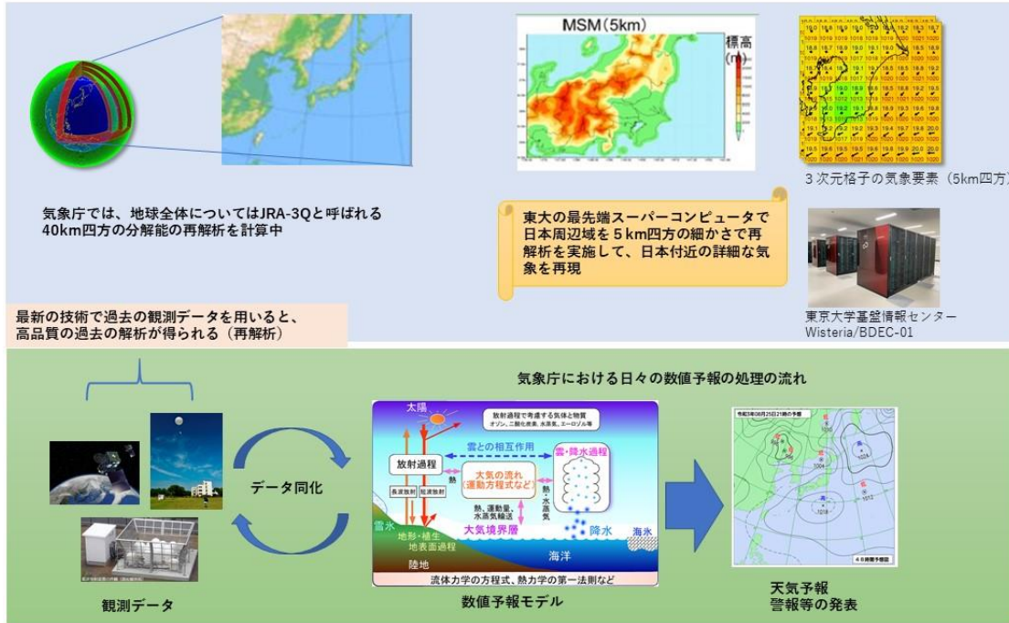
図1：日本域気象再解析とは
