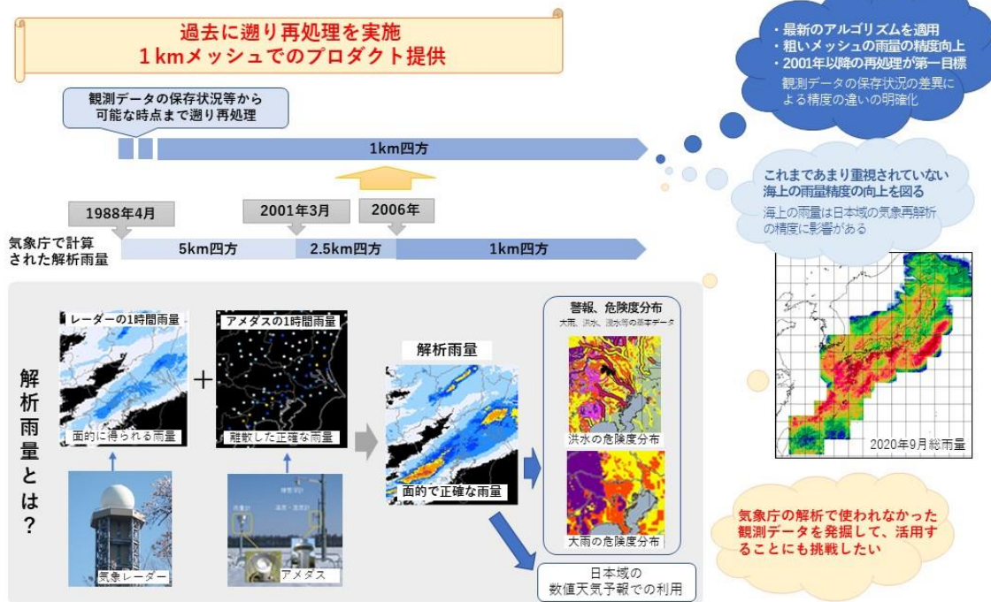
図2：過去の解析雨量の再処理概要
